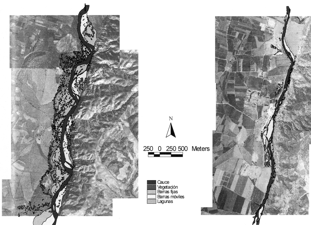
Figura 2. Evolución de la dinámica fluvial del río a la altura del Soto de la Chopera, entre 1956 y 1999. En 1956, la anchura del cinturón de meandros coincide con la sección determinada por las barras fijas y móviles, y existen paleocauces en la llanura de inundación indicativos de un río con dinámica propia y gran actividad. En 1999, se ve que el río ha perdido prácticamente todo el espacio con que contaba, con lo cual no puede expandirse lateralmente y esto genera unos problemas de incisión y también la disminución de la anchura del cauce. Este encajamiento y rectificación es debido una vez más al cambio de usos del suelo asociado al terreno fluvial, que han sido ocupados por cultivos o graveras a ambos lados del Jarama haciendo inexistente el terreno asociado al cauce, y esto hace aumentar los fenómenos de erosión y la inestabilidad de las orillas. Evolution of fluvial dynamics of the river Jarama at Soto de la Chopera between 1956 and 1999. In 1956, the meander belt width was about equal the section defined by mobile and steady bars. Also, there were a number of palaeochannels in the floodplain, indicative of a river with active dynamics. In 1999, the river had almost lost its entire floodplain and thus could not expand laterally, causing incision of the channel with consequent decreases in channel width. Floodplain encroachment and rectification has been caused by changes in land use. Floodplain areas on both banks have been occupied by gravel minings and agricultural activities, increasing erosion and instability of the channel banks.
