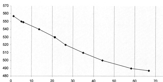
Figura 1. Perfil longitudinal del río Jarama a su paso por el Parque Regional del Sureste. Longitudinal profile of the Jarama River (Spain) within the Southwest Regional Park.
